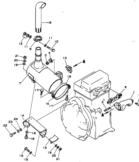
エキゾーストマニホールドおよびマフラー FIG. 121 EXHAUST MANIFOLD AND MUFFLER
