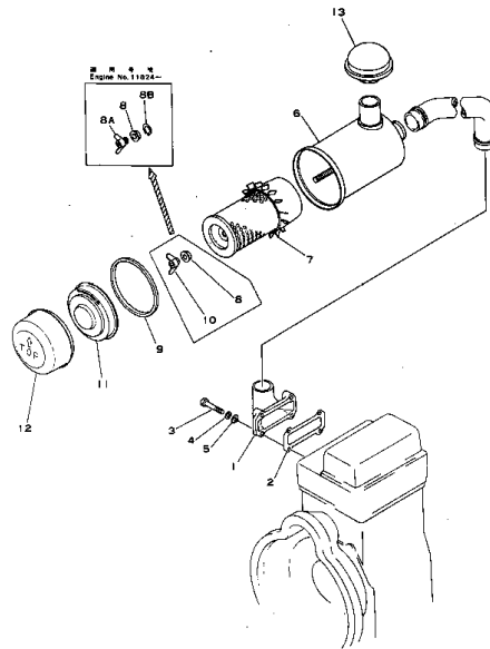
エアークリーナとエアーインテークマニホールド FIG. 111 AIR INTAKE MANIFOLD AND AIR CLEANER
