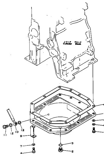
オイルパン FIG. 215 OIL PAN
