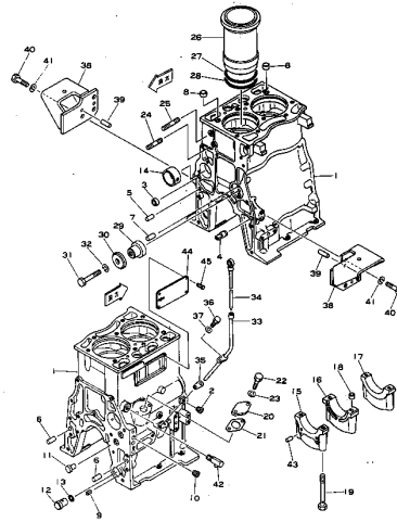
シリンダブロック FIG. 201 CYLINDER BLOCK
