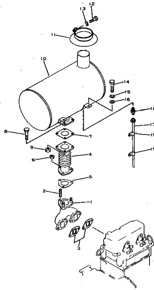
エキゾースト マニホールド および マフラー Fig. 124 EXHAUST MANIFOLD AND MUFFLER ( 通用 号 機 EG15S Engine No. 17329~ )
