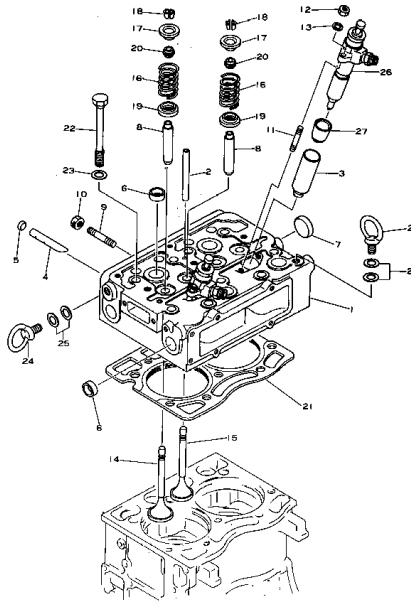
シリンダ ヘッド Fig. 101 CYLINDER HEAD
