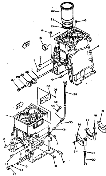
シリンダブロック (EG15 Engine No. 16977~) Fig. 202 CYLINDER BLOCK (EG15S Engine No. 17329~)
