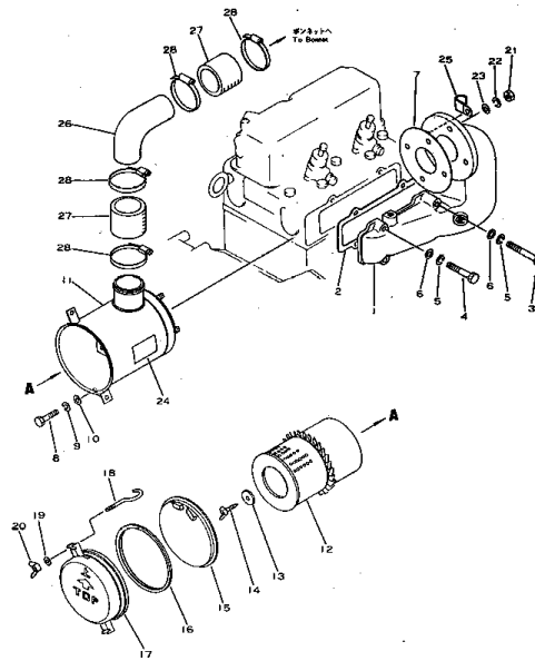
インテーク マニホールド および エアークリーナ Fig. 112 INTAKE MANIFOLD AND AIR CLEANER (適用 号 機 (EG15S Engine No. 17329~))
