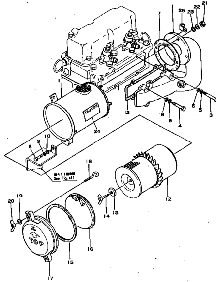
インテーク マニホールド および エアークリーナ Fig. 111 INTAKE MANIFOLD AND AIR CLEANER (D10 Engine No. 11225~) (PC02 Engine No. 16531~) (EG15 Engine No. 16977~)
