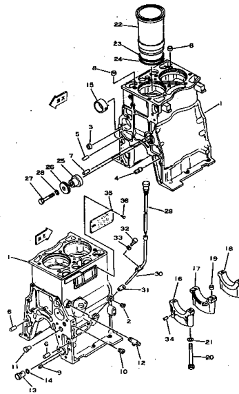
シリンダブロック (EG15 適用号機) Fig. 202 CYLINDER BLOCK (EG15 Engine No. 16977~) (EG15S Engine No. 17329~)
