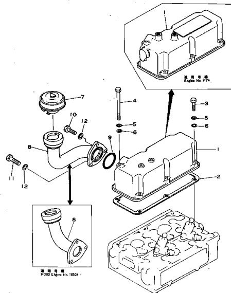
シリンダヘッドカバー Fig. 105 CYLINDER HEAD COVER
