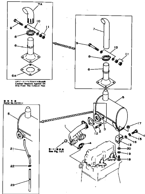
エキゾースト マニホールド および マフラー Fig. 122A EXHAUST MANIFOLD AND MUFFLER (適用 号 数 (PC 02 Engine No. 20028~))
