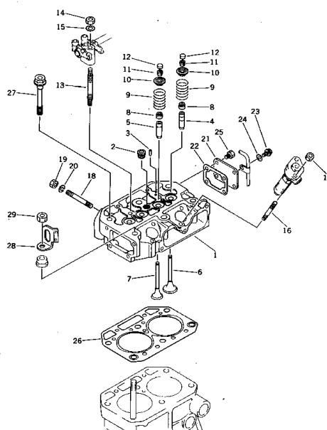
シリンダヘッド Fig. 101 CYLINDER HEAD
