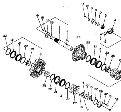
ドライブタンブラ Fig. 307 DRIVE TUMBLER
