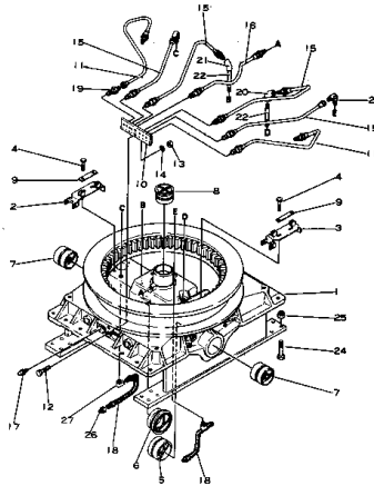
トラック フレーム および ルーブリケーティング パイピング Fig.302 TRUCK FRAME AND LUBRICATING PIPING (25-BSC)
