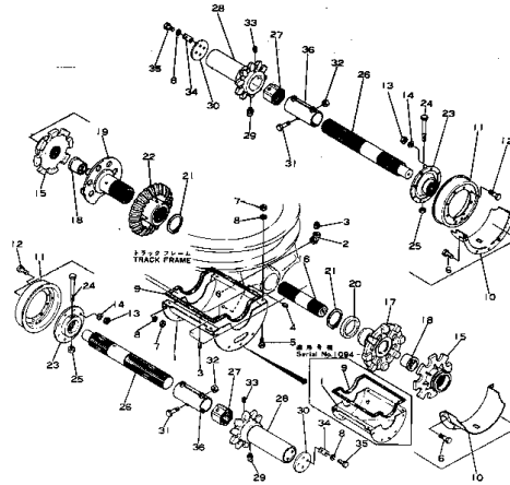
プロペル ★リソソナル シャフト Fig.230 PROPEL HORIZONTAL SHAFT (25-BSC)
