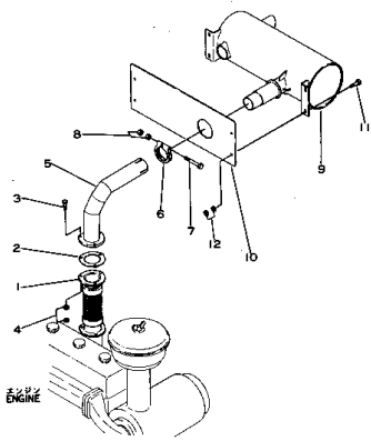
Fig.102 エキゾーストライン (機番 1001～1093) EXHAUST LINE (Serial No.1001～1093)
