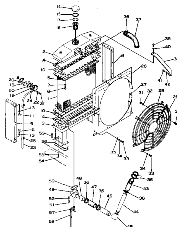
Fig. 103 RADIATOR
