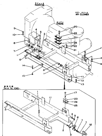
Fig.101 エンジン取り付け部品 (Serial No.1001~1093)
