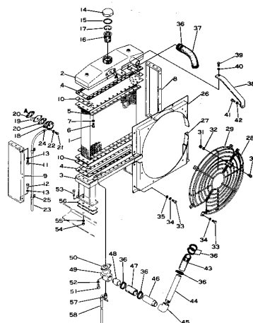
Fig. 103 RADIATOR
