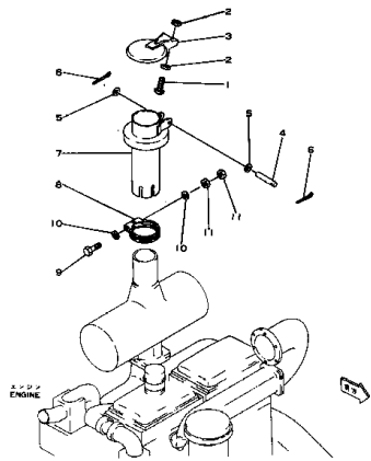
Fig. 103 エキゾースト パイプ EXHAUST PIPE (22-BCM Serial No. 1001~1044, 1047~1063) (22-BHD Serial No. 1001~1005)
