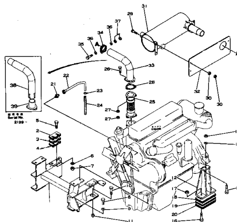
エンジン取付部品 および エキゾースト パイプ Fig. 101B ENGINE ATTACHING PARTS AND EXHAUST PIPE (適用 号機 Serial No. 2001~)
