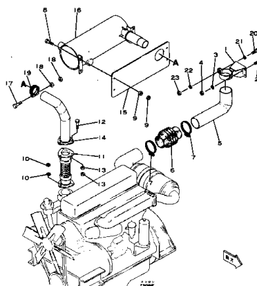
Fig. 103B エキゾーストパイプ EXHAUST PIPE (22-BCM Serial No. 1143~1220) (22-BHD Serial No. 1018~1035)
