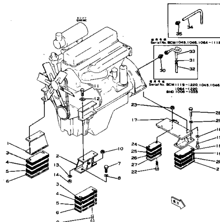
エンジン取付部品 Fig. 101A ENGINE ATTACHING PARTS (22-BCM Serial No. 1045, 1046, 1064~1220) (22-BHD Serial No. 1006~1035)
