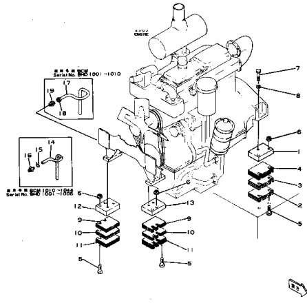
エンジン取付部品 Fig. 101 ENGINE ATTACHING PARTS (適用機種 22-BCM Serial No. 1001~1044, 1047~1063) (22-BHD Serial No. 1001~1005)
