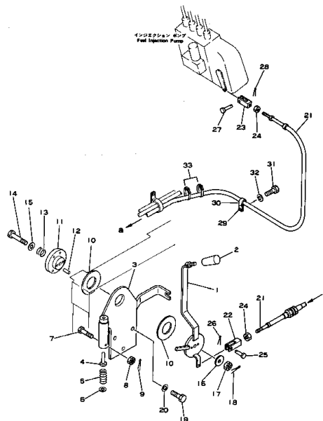
Fig. 1121 フュエル コントロール レバー 取付け リンケージ FUEL CONTROL LEVER AND LINKAGE
