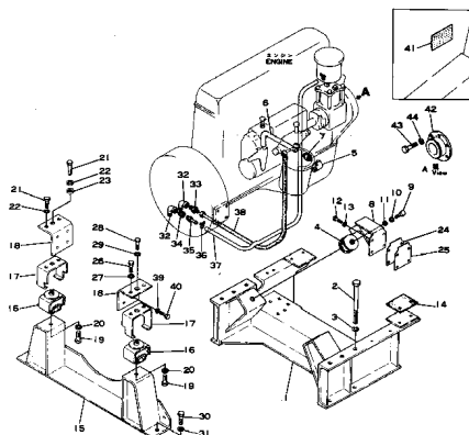
Fig. 101 エンジン サポート (適用 号機 (Serial No. 1003~1008))
