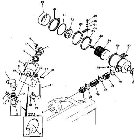
Fig. 102A エアー インテーク および エキゾースト ライン (適用 機種 Serial No. 1287 ~)
