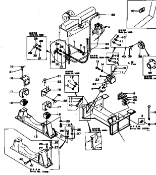
エンジン サポート (図 101A) (Serial No. 1009~)
