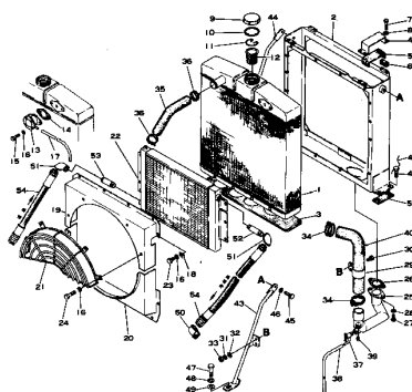
Fig. 103 クーリング システム (適用 号 機 COOLING SYSTEM (Serial No. 1003~1065) (1111A, 1128A, 1138A 1168A, 1196A, 1132B)
