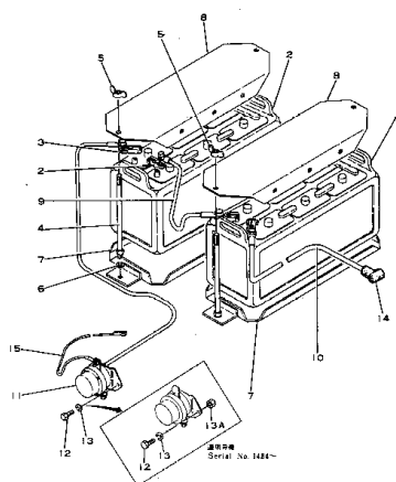
バッテリー および リレー スイッチ Fig. 106 BATTERY AND RELAY SWITCH
