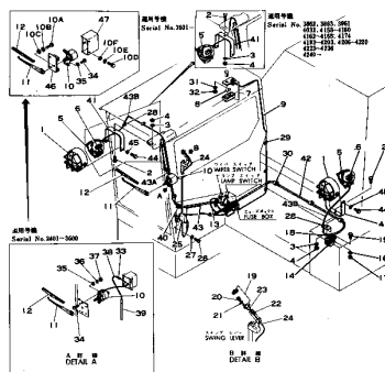
電 氣 系 統 (適用年表) Fig. 107A ELECTRICAL SYSTEM (Serial No. 2401~)
