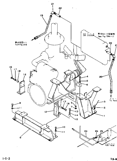
エンジン 取付部品 Fig. 101A ENGINE ATTACHING PARTS, オイルクーラおよびフエエルライン (適用機種 OIL COOLER AND FUEL LINES (Serial No. 5001~)
