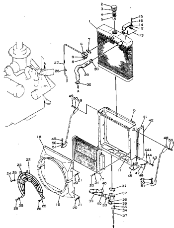
ラジエータ (■●●●●) Fig. 104 A RADIATOR (Serial No. 5001~)
