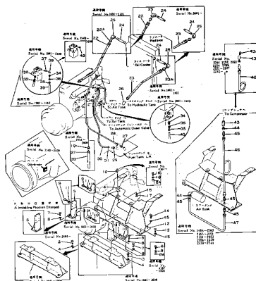
エンジン 取付 図 Fig. 101 ENGINE ATTACHING PARTS. オイルクーラ及び燃料ライン (適用機種 OIL COOLER AND FUEL LINE (Serial No. 1001-5000)
