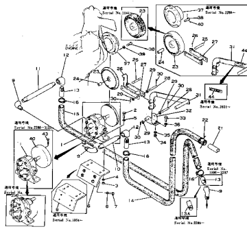
燃料給油装置(適用号機) Fig. 105 FUEL FILLER SYSTEM (Serial No. 1001~5000)
