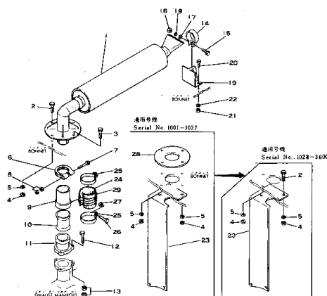
エキゾースト マフラー (通用仕様) Fig. 103 EXHAUST MUFFLER (Serial No. 1001~3600)
