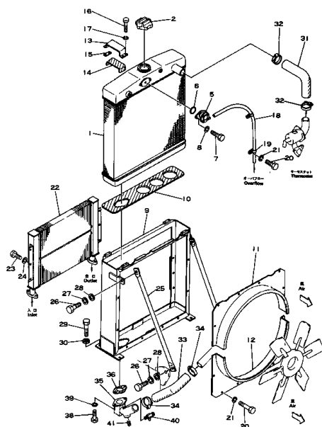
ラジエータ および オイル クーラ Fig. 103 RADIATOR AND OIL COOLER
