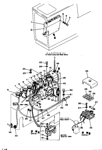
Fig. 107 インストルメント パネル および エレクトリカル システム INSTRUMENT PANEL AND ELECTRICAL SYSTEM
