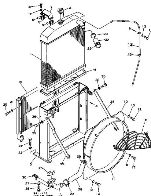
Fig. 1131 ラジエーター および オイルクーラー RADIATOR AND OIL COOLER
