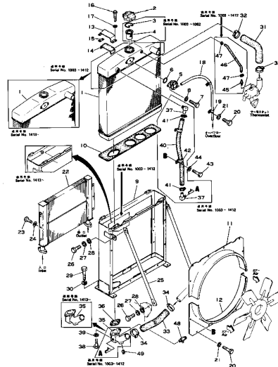
Fig. 103 ラジエーター および オイル クーラー RADIATOR AND OIL COOLER
