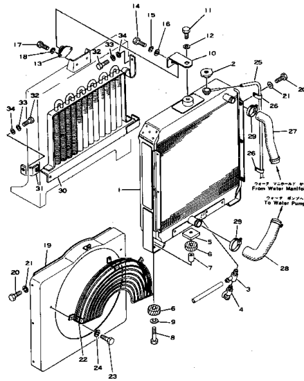
ラジエータ および オイル クーラ Fig. 1131 RADIATOR AND OIL COOLER
