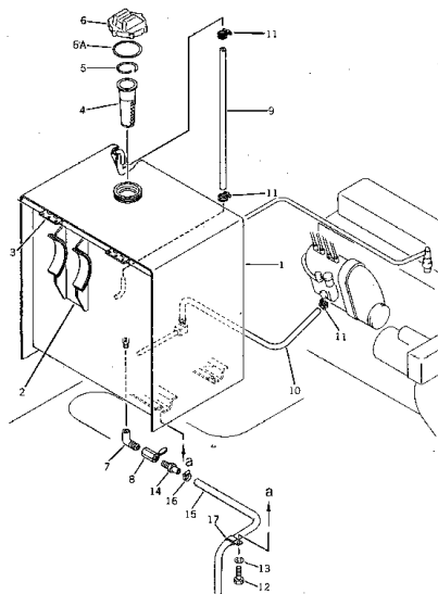
Fig. 1141 フUEL タンク 及び パイピング FUEL TANK AND PIPING
