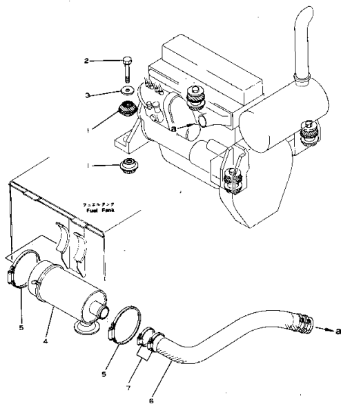
エンジン 取付 部品 Fig. 1101 ENGINE ATTACHING PARTS
