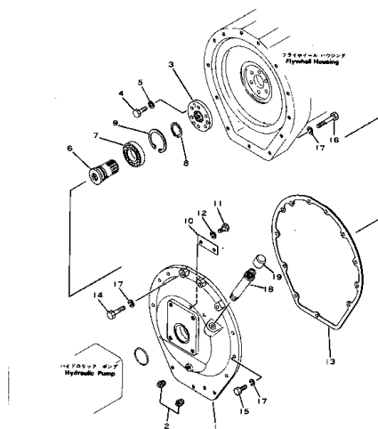
パワー タイク オフ Fig. 1105 POWER TAKE OFF
