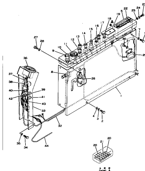
インストルメント パネル Fig. 1155 INSTRUMENT PANEL
