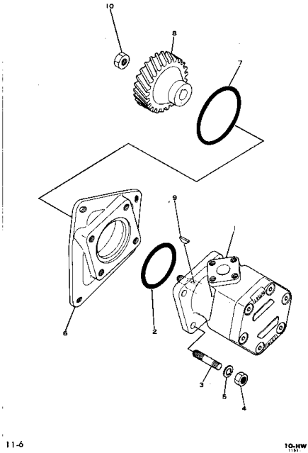
パワーテイク オフ (ステアリング ポンプ用) Fig. 1106 POWER TAKE OFF (For Steering Pump)
