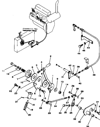
Fig. 1121 フューエル コントロール レバー および リンケージ FUEL CONTROL LEVER AND LINKAGE 適用 号 数 10-HT Serial No. 6001 ~ 9500 10-HQ Serial No. 6001 ~ 8616 10-HL Serial No. 6001 ~ 6200
