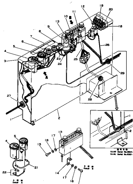
Fig. 1155 インスツルメント パネル INSTRUMENT PANEL
