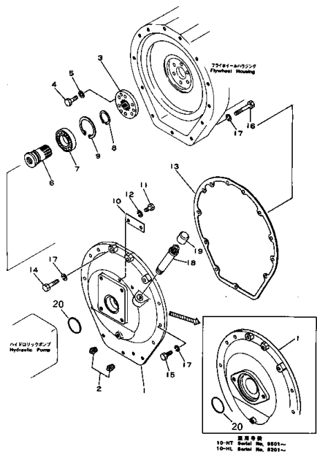
Fig. 1105 パワー テイク オフ POWER TAKE OFF
