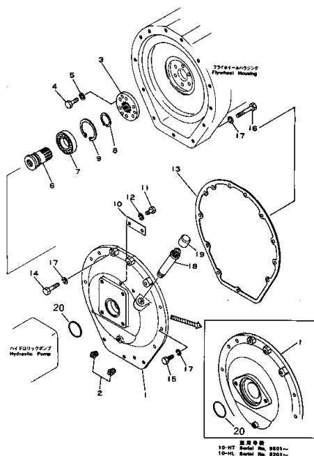
Fig. 1105 パワー テイク オフ POWER TAKE OFF
