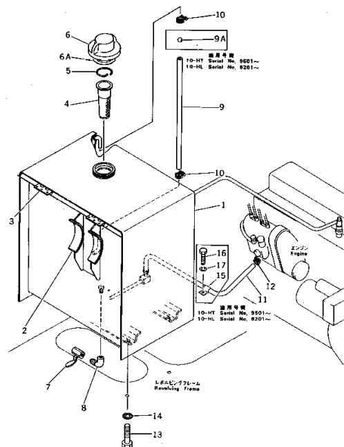
Fig. 1141 フュエル タンク および パイピング FUEL TANK AND PIPING
