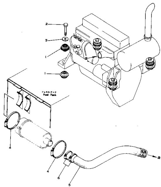
Fig. 1101 エンジン マウント ENGINE MOUNT
