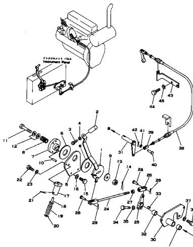
Fig. 1121 フューエル コントロール レバー および リンケージ FUEL CONTROL LEVER AND LINKAGE
