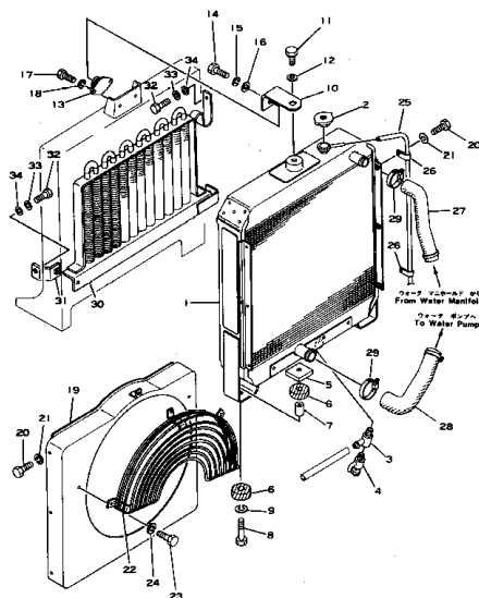
ラジエータ および オイル クーラ Fig. 1131 RADIATOR AND OIL COOLER
