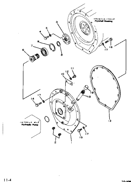
パワー タイク オフ Fig. 1105 POWER TAKE OFF
