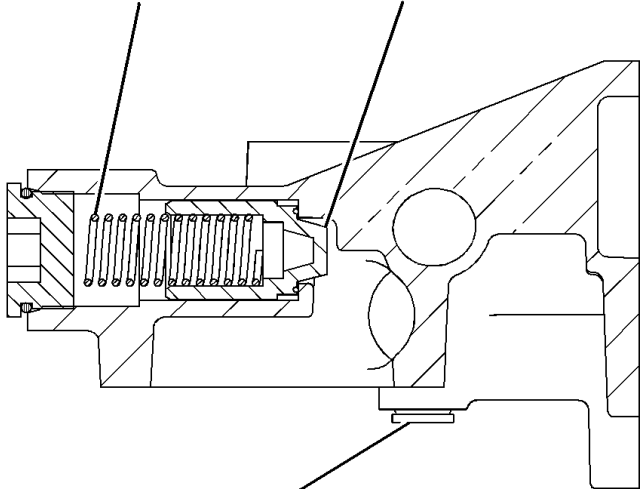
SECTION D-D
