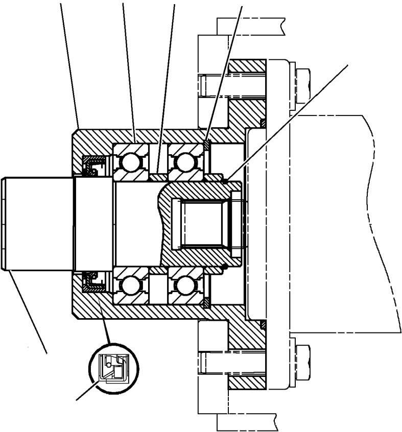
SECTION A-A
