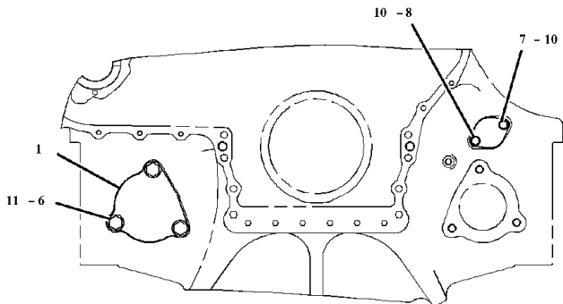
VIEW A-A
