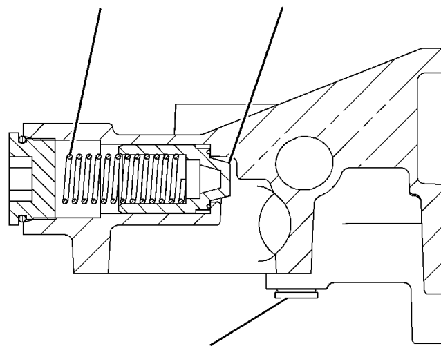
SECTION D-D
