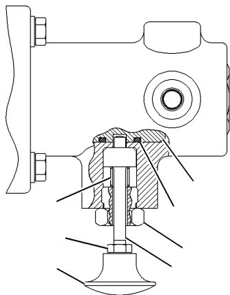
VIEW A-A
