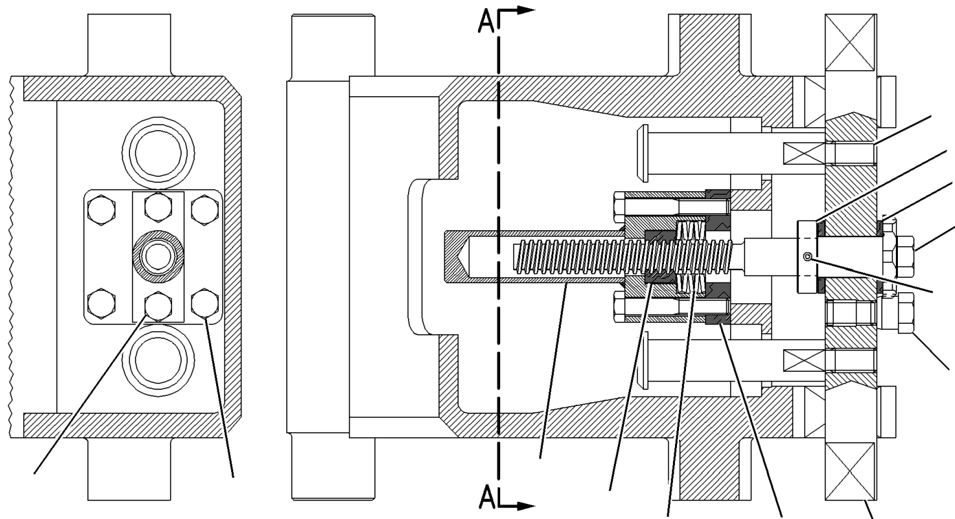
SECTION A-A
