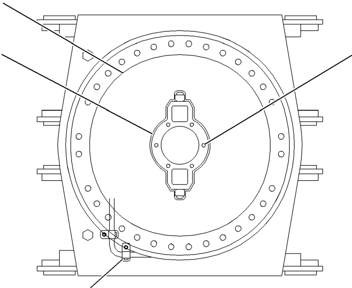
VIEW A-A
