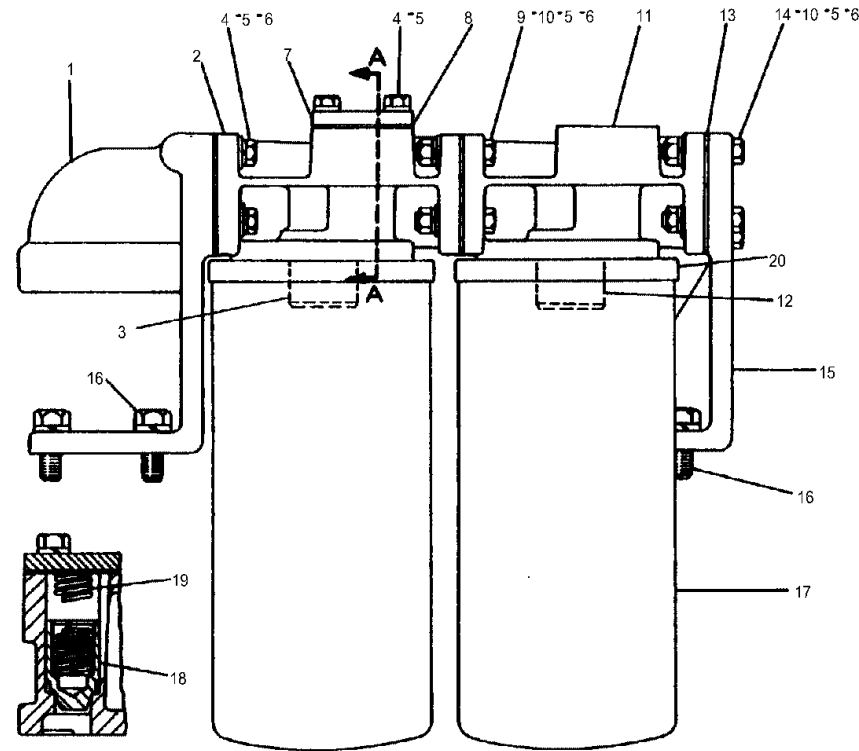
SECTION A-A
