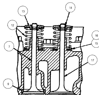
VIEW A-A
