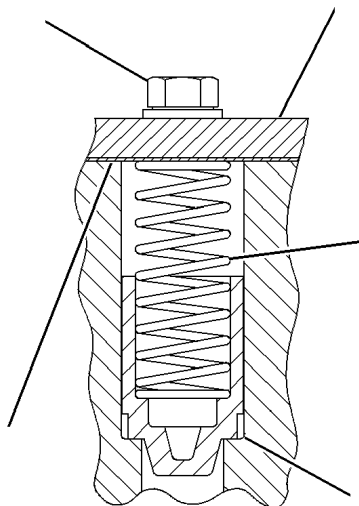
VIEW A-A
